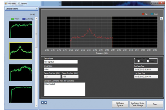
Abbildung 4: Automatische Erkennung aller HF-Störungsquellen
