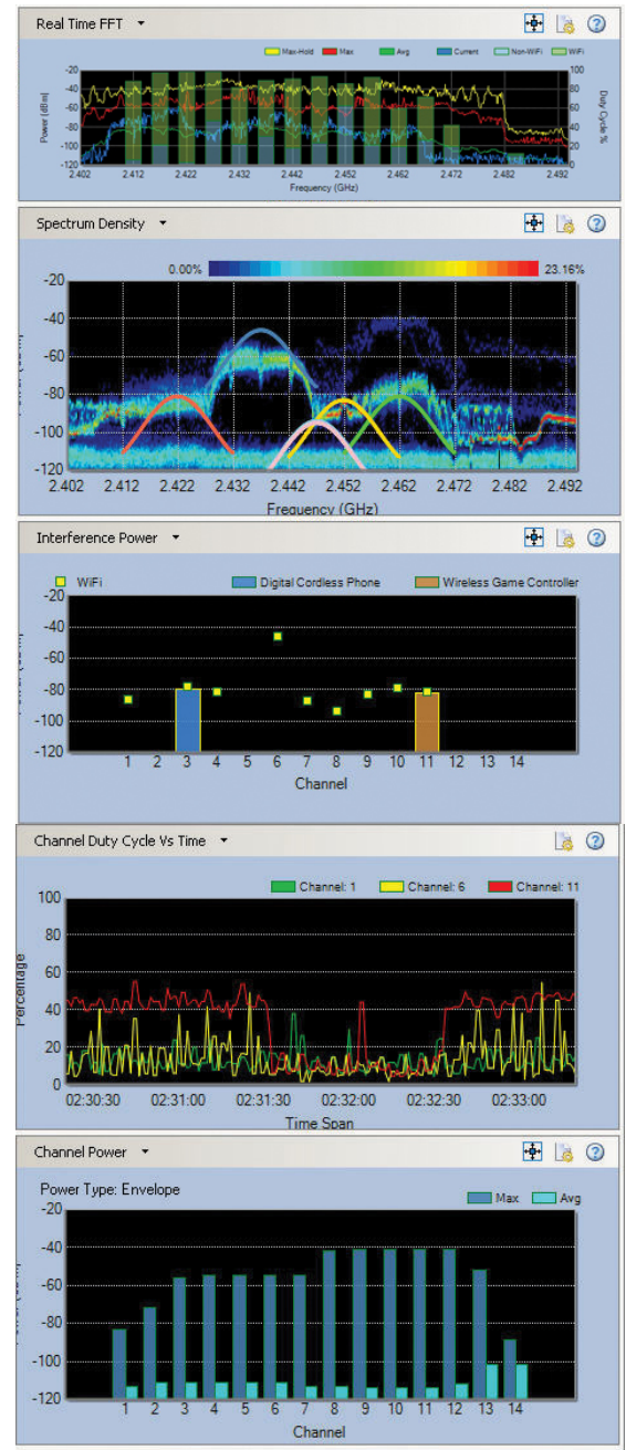
Abbildung 1: HF-Spektraldiagramme
