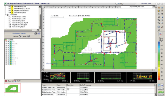
Abbildung 6: Integration mit AirMagnet Survey
